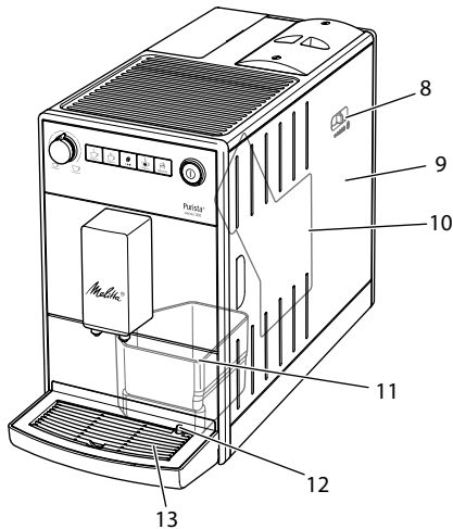
Att. 2: lerīce no priekšpusēs, labā puse
